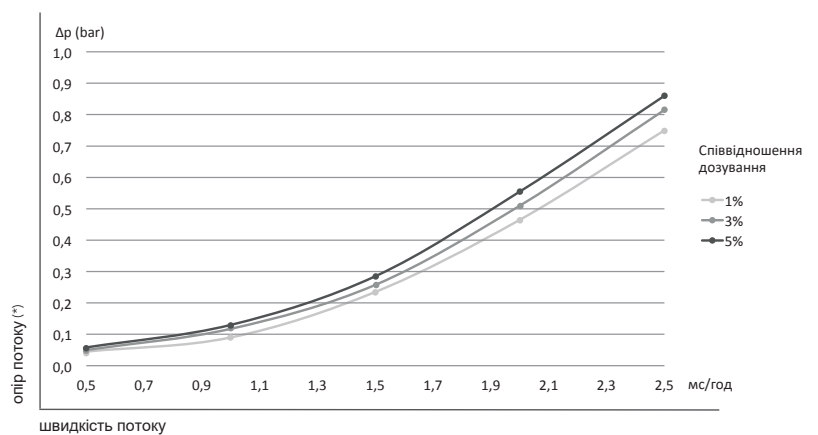
Графік опору потоку - дозатора 1 - 5 %
