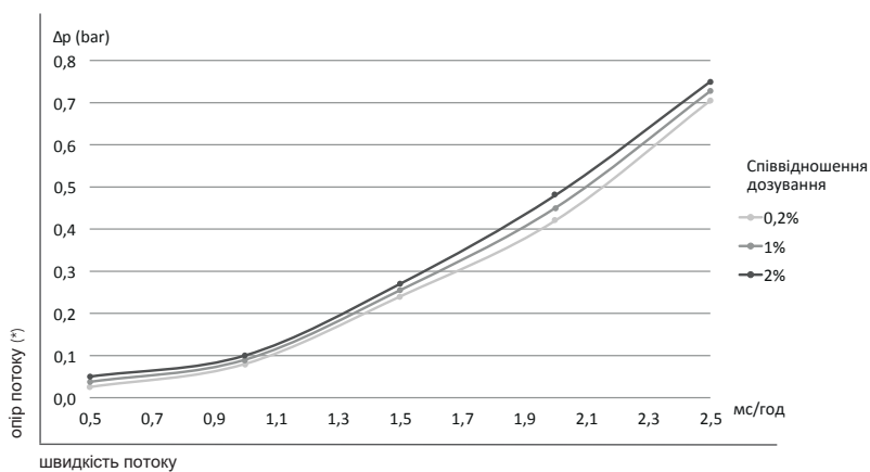
Графік опору потоку - дозатора 0,2%-2%
